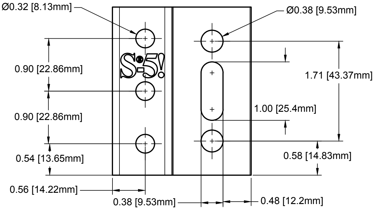
Top
